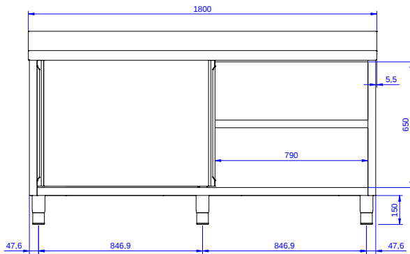
Alzado
